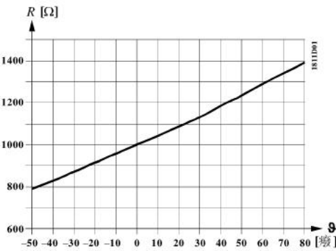
特性 LG-Ni 1000
